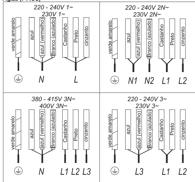
Fig.2b (7 FIOS)
