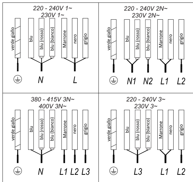
Fig.2b (7 FILI)
