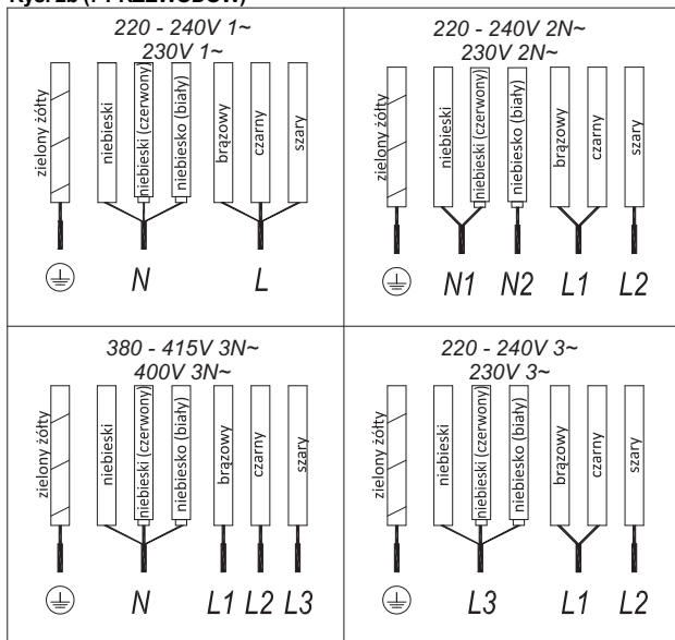
Rys. 2b (7 PRZEWODÓW)
