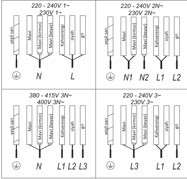
Şekil 2b (7 KABLO)
