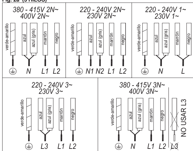
Fig. 2a (5 HILOS)
