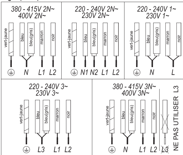
Fig.2a (5 FILS)
