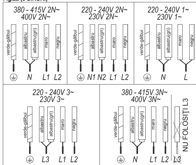
Fig.2a (5 SIRURI)
