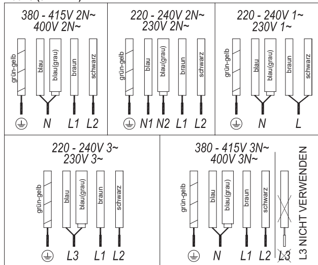
Abb.2a (5 KABEL)
