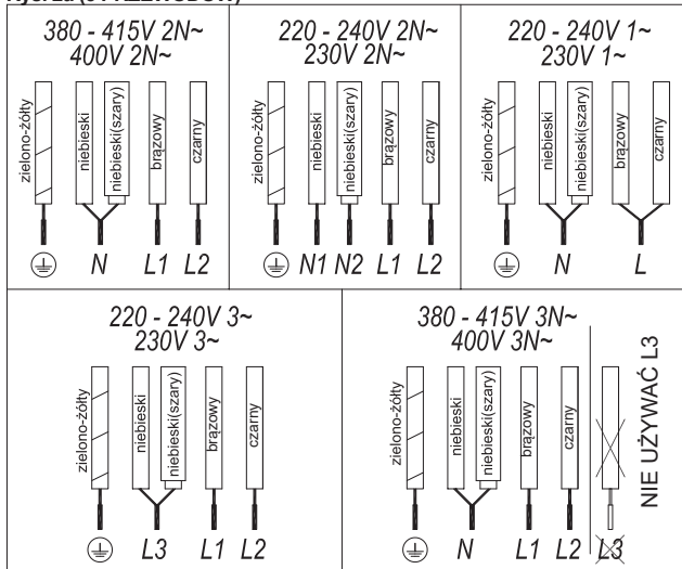
Rys. 2a (5 PRZEWODÓW)
