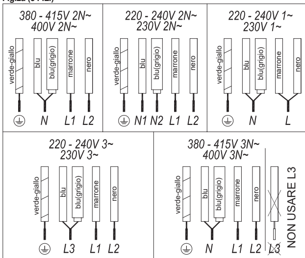
Fig.2a (5 FILI)
