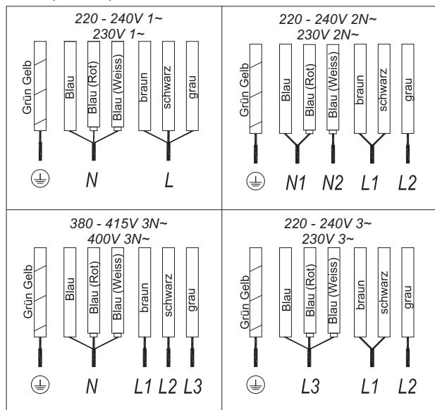
Abb.2b (7 KABEL)
