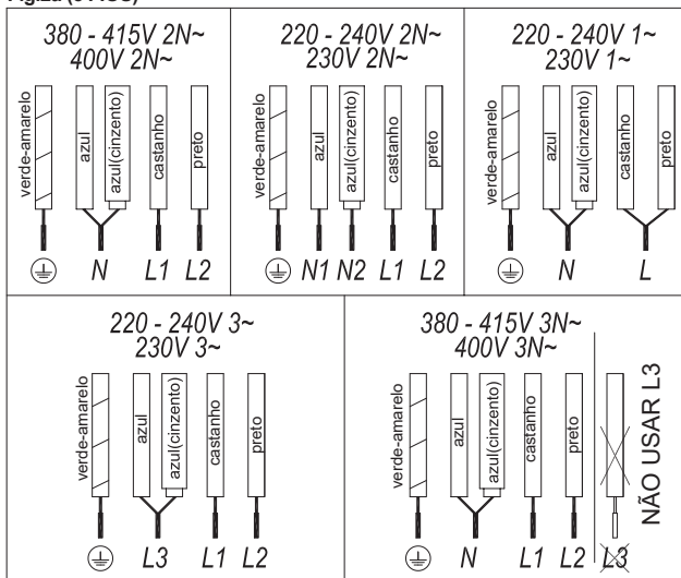
Fig.2a (5 FIOS)
