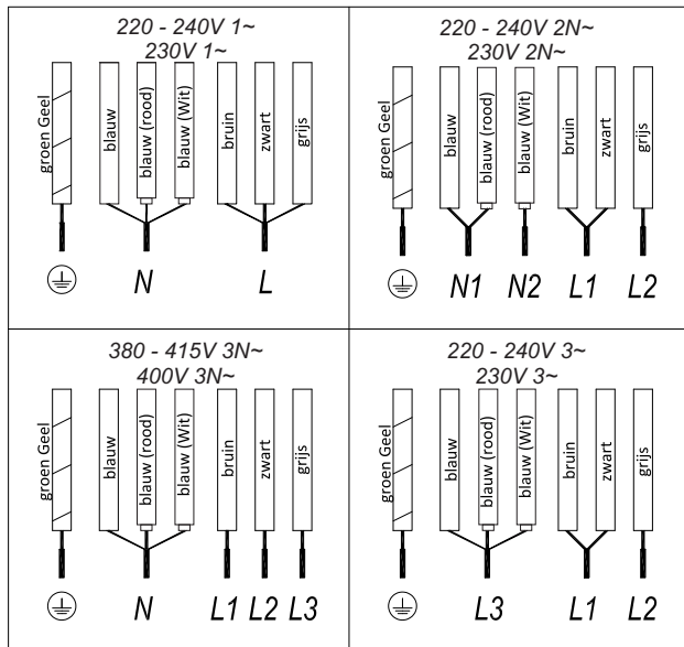
Afb. 2b (7 DRADEN)
