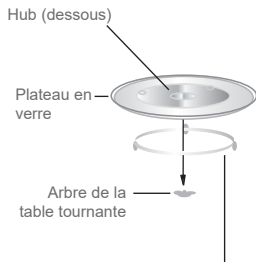
Assemblage d'un anneau de plateau tournant
