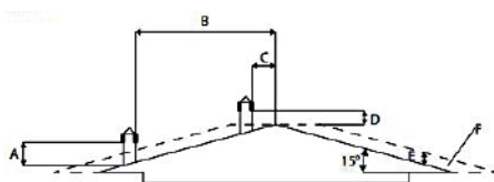
TETO A 15°
