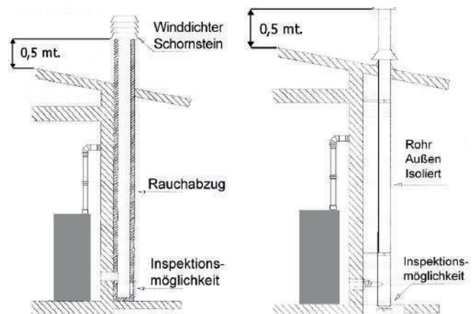
Abb. 2: Anschluss an den Rauchabzug
