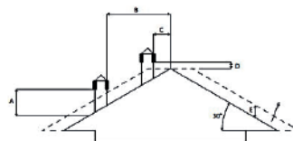
TECHO DE 30°
