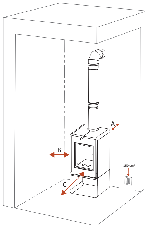
A) Distância mínima à retaguarda 50 cm B) Distância lateral mínima de 40 cm C) Distância mínima à frente 120 cm
