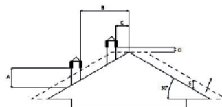
TOIT À 30°
