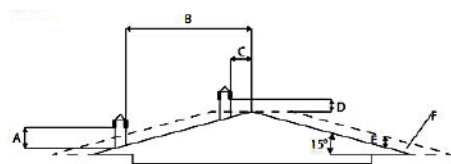
15° DAK
