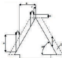
TECHO DE 60°
